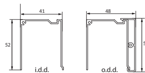
U-profiel (bovengeleider)
