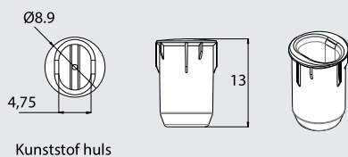
Kunststof huls
